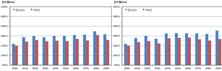
그림 3-4. 경상남도와 거창군의 연강수량(mm) 시계열 (RCP4.5(좌), RCP8.5(우))
