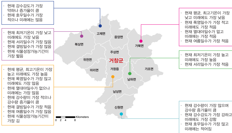
그림 5-1. 경상남도 거창군의 읍면별 기후변화 전망 요약
