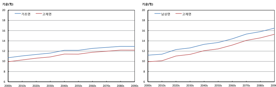
그림 3-2. 평균기온(℃) 증가율이 가장 큰 지역(고제면)과 작은 지역(가조면, 남상면)의 시계열(RCP4.5(좌), RCP8.5(우))
