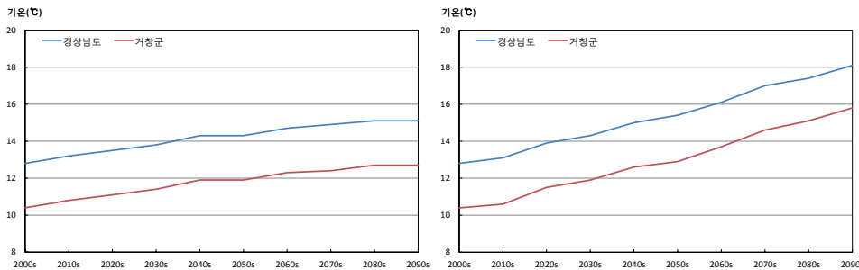
그림 3-1. 경상남도과 거창군의 평균기온(℃) 시계열(RCP4.5(좌), RCP8.5(우))
