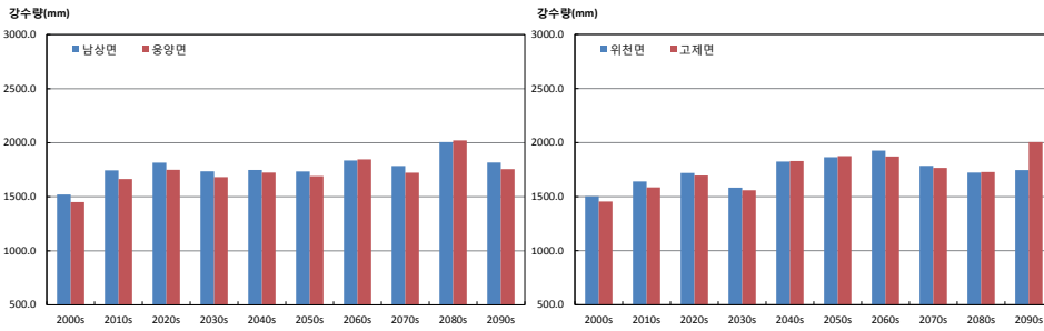
그림 3-5. 연강수량(mm) 증가율이 가장 큰 지역 (웅양면, 고제면)과 작은 지역(남상면, 위천면)의 시계열 (RCP4.5(좌), RCP8.5(우))
